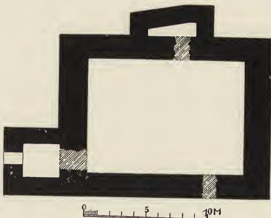
Fig. 180. Mahlitzsch, Burgruine. Grundriss.
